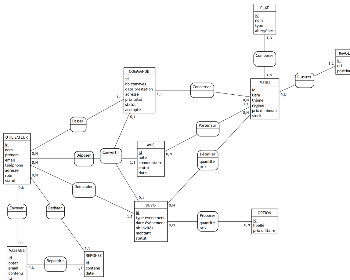
Figure 2 — Modèle Conceptuel de Données (MCD)
